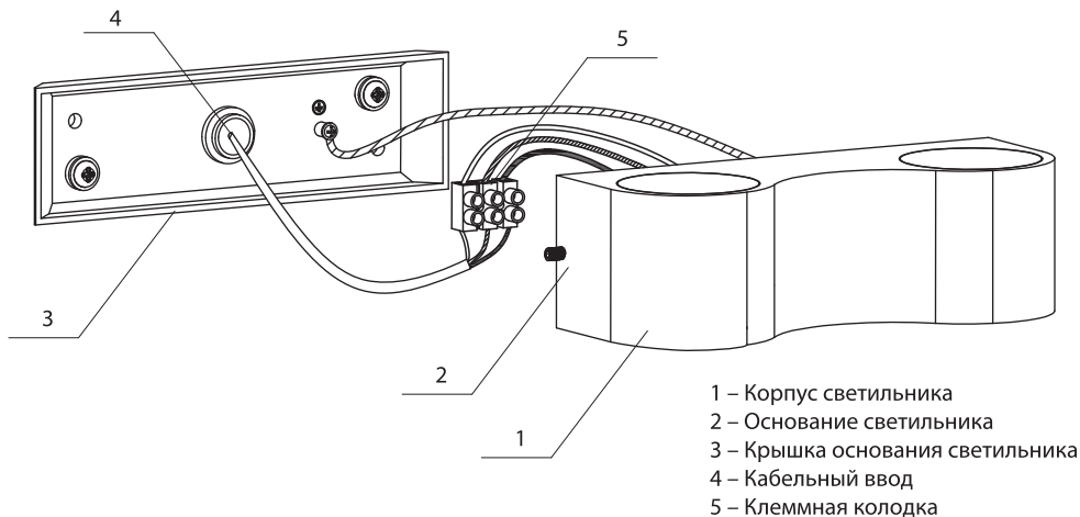
Рисунок 1. Конструкция светильника
